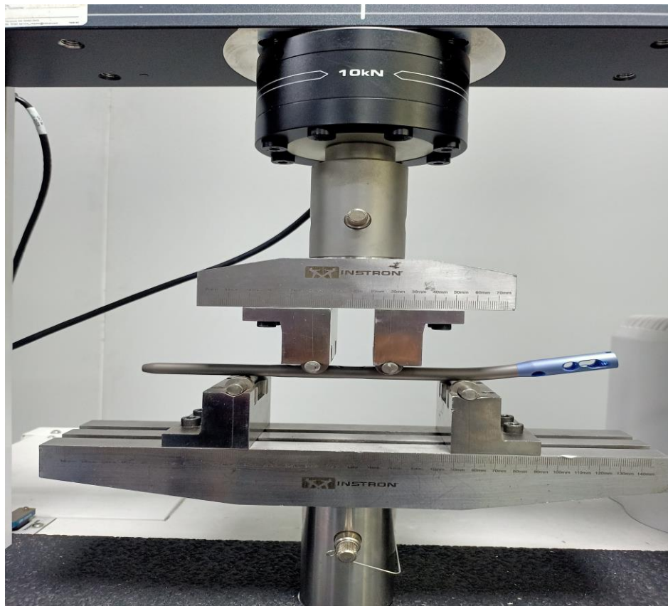
Fig: Test Setup
