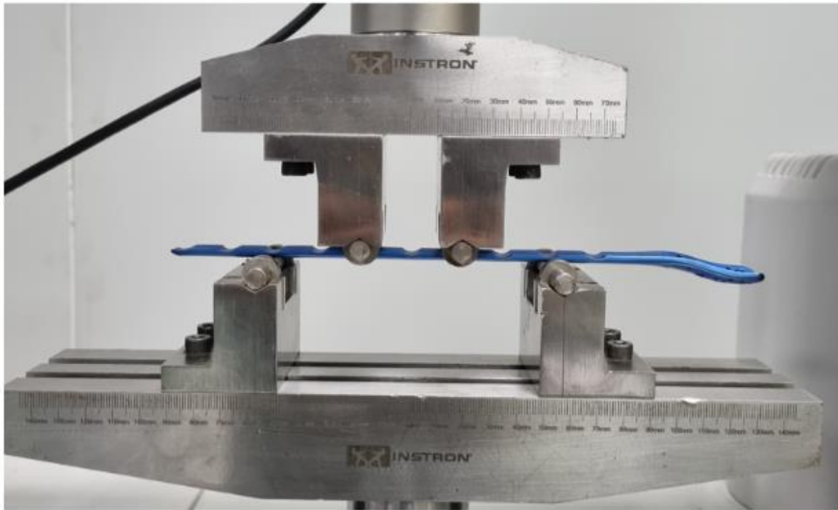
Fig: Test Setup
