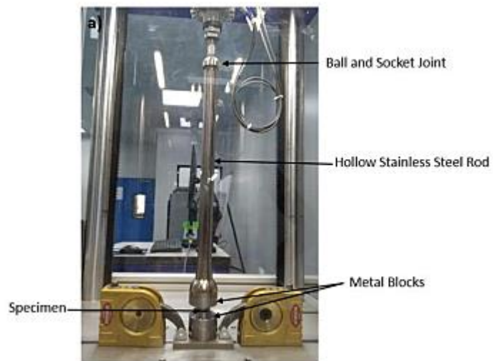
Fig: Test Setup
