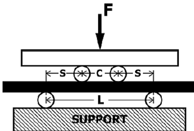
fig: Test Setup
