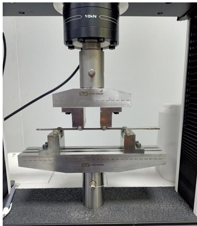
fig: Test Setup
