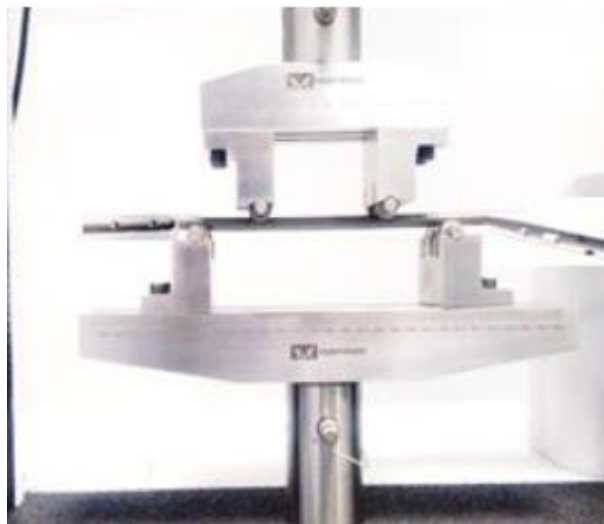
Fig: Test Setup
