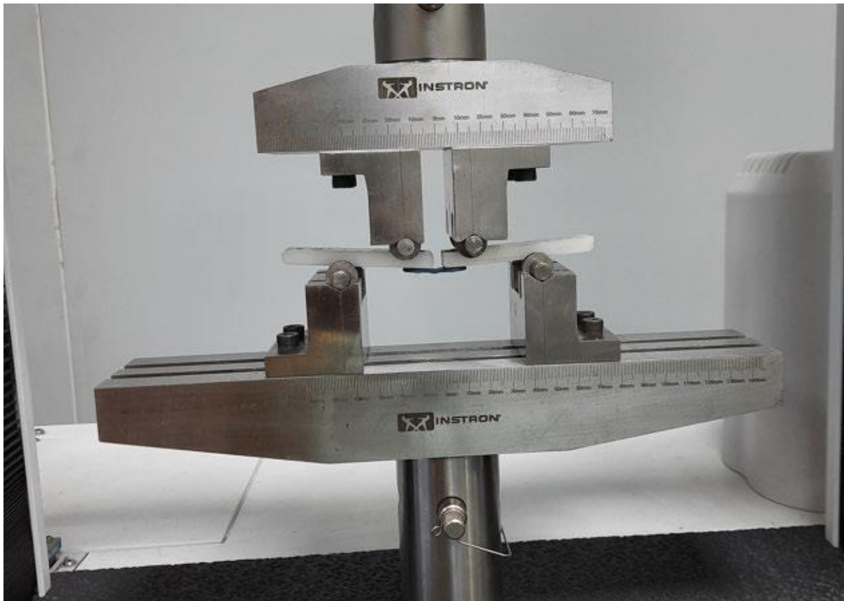
Fig: Test Setup
