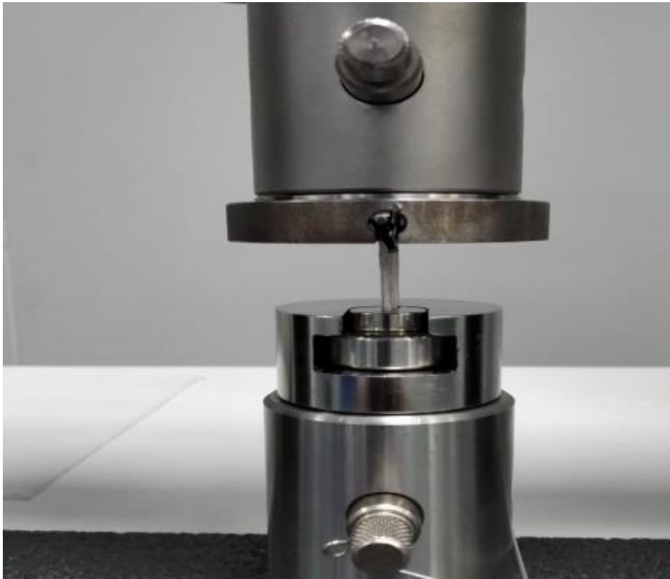
Fig: Test Setup
