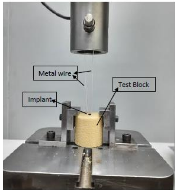
Fig: Test Setup
