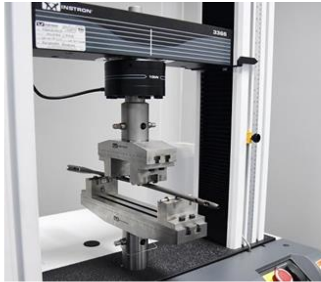
Fig: Test Setup
