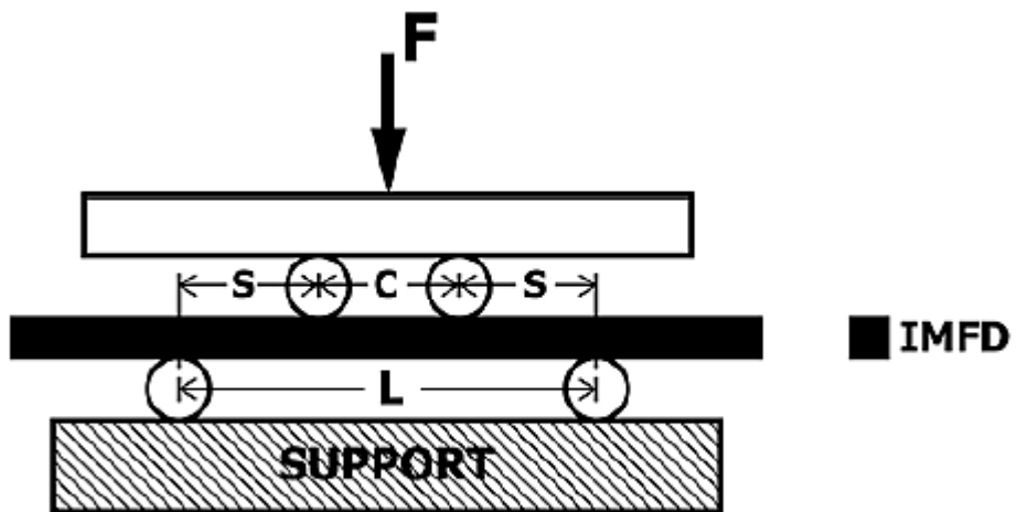
Fig: Test Setup
